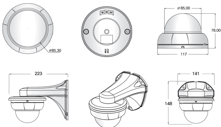
STAFFA DI FISSAGGIO A PARETE art. 7707-WALL-D100
