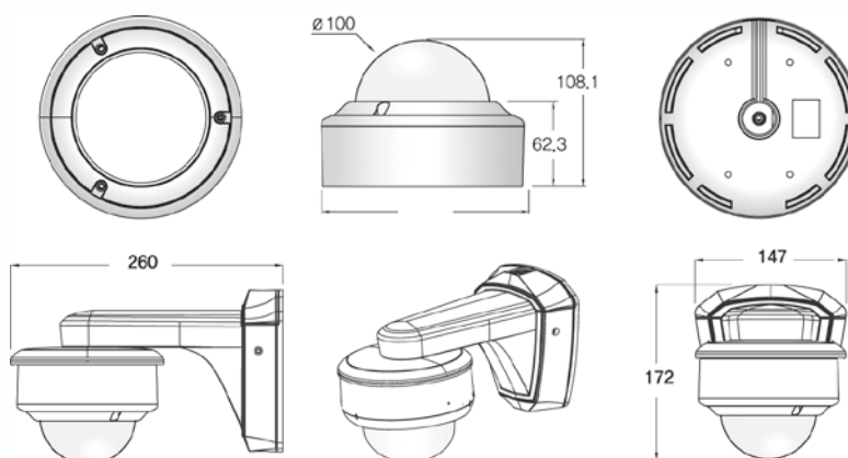
STAFFA DI FISSAGGIO A PARETE art. 7704-WALL-V100
